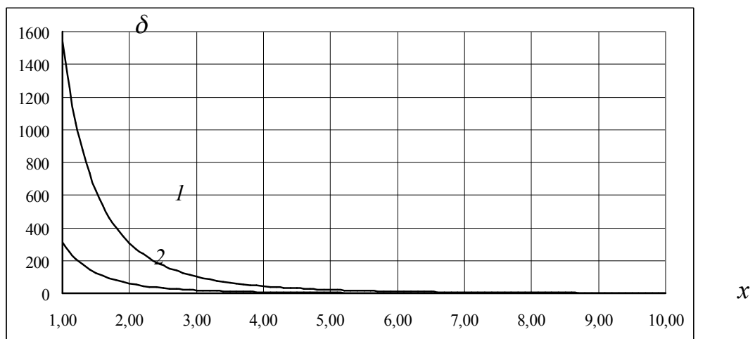
Рис. 2.12. Графіки відносної похибки екстраполяції за нижню межу навчальних даних
