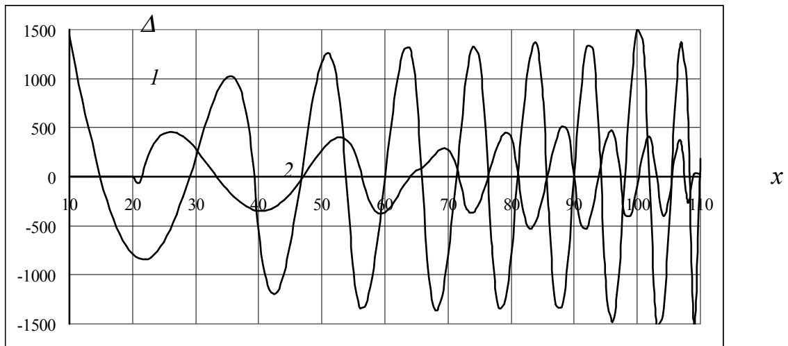
Рис. 2.7. Графіки абсолютної похибки навчання
