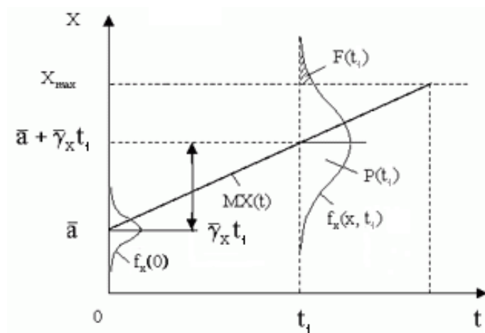
Рис. 2.2. Графічне зображення моделі ПК
