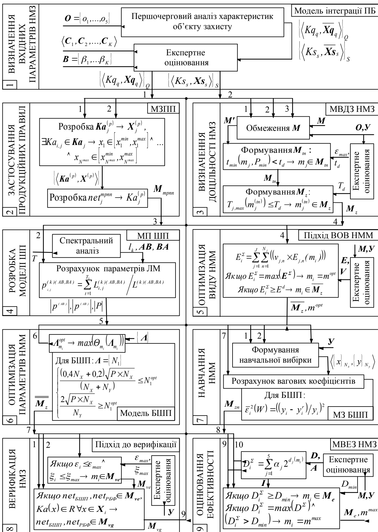
Рис. 4.6. Схема методології неймережевого оцінювання ПБ
