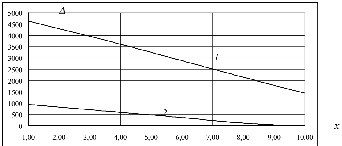
Рис. 2.11. Графіки абсолютної похибки екстраполяції за нижню межу навчальних даних
