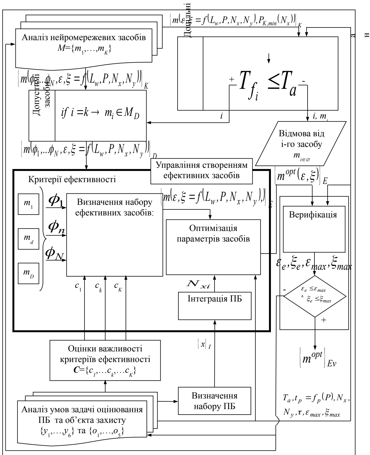
Рис. 3.11. Модель процесу створення ефективних НМЗ виявлення кібератак
