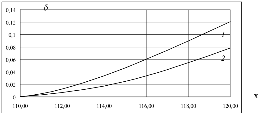
Рис. 2.10. Графіки відносної похибки екстраполяції за верхню межу навчальних даних
