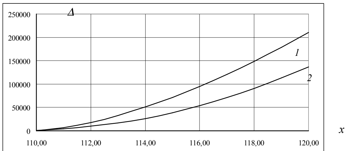
Рис. 2.9. Графіки абсолютної похибки екстраполяції за верхню межу навчальних даних
