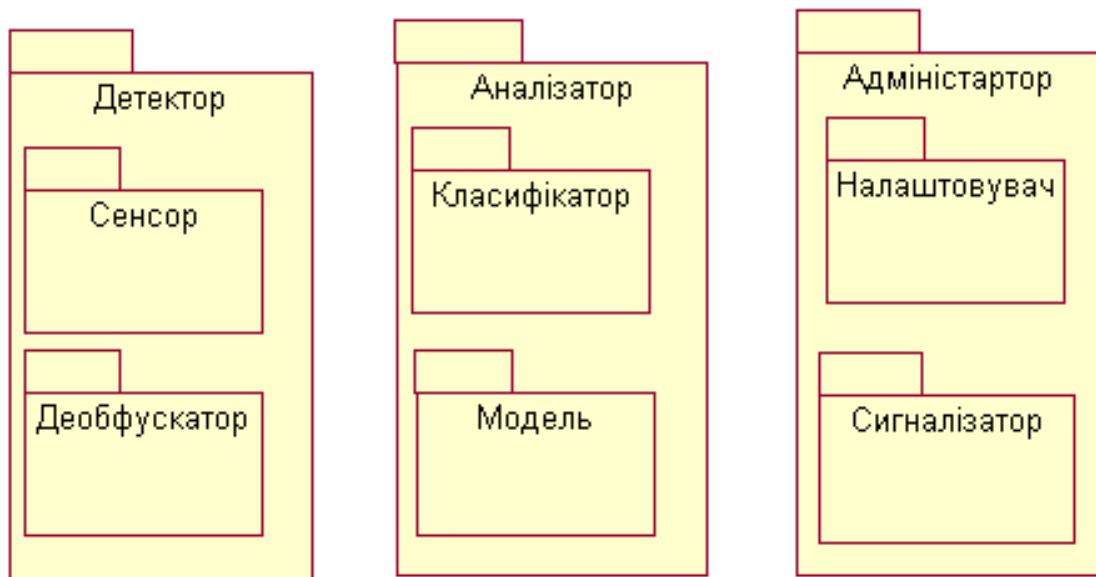
Рис. 4.2. Діаграма пакетів
