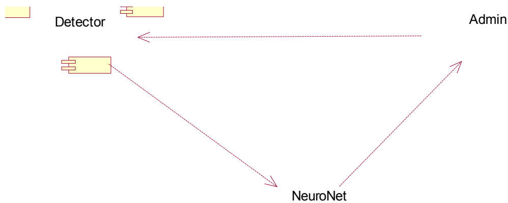
Рис. 4.3. Діаграма компонентів
