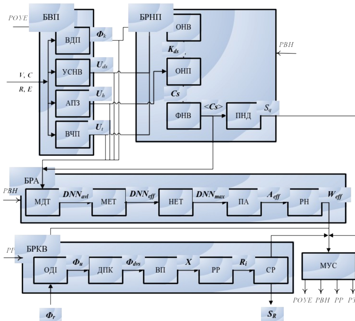
Рис. 4.6. Структура нейромережевої системи розпізнавання комп'ютерних вірусів
