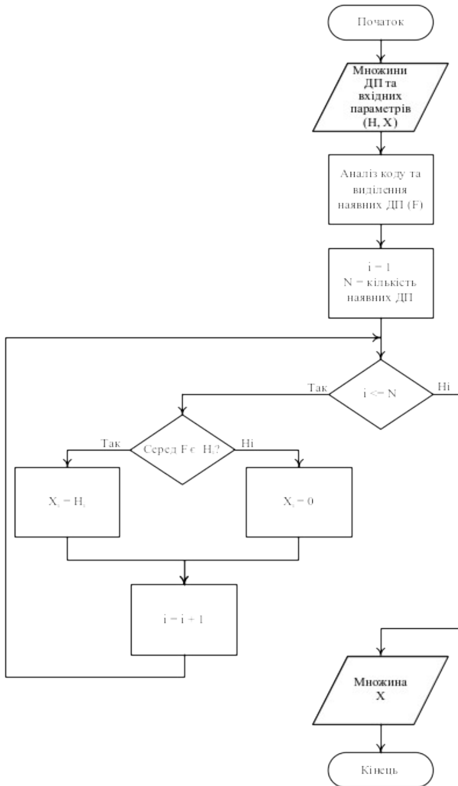
Рис. 4.9. Структура алгоритму формування вхідного шару ГНМ
