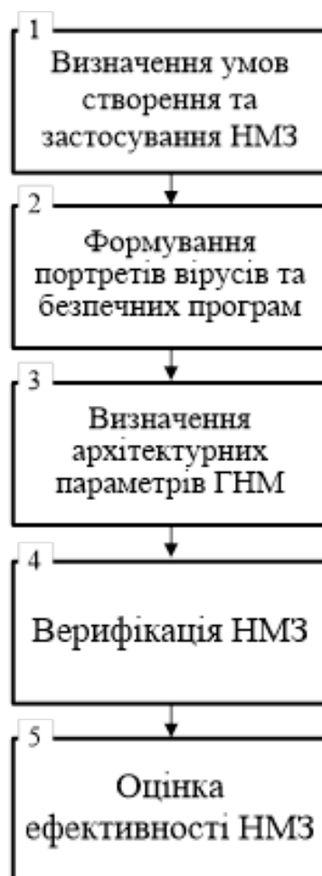
Рис. 3.14 Структурна схема методу нейромережевого розпізнавання вірусів
