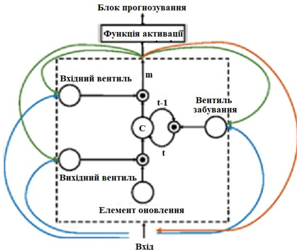
Рис. 1.2.5. Структурна схема блоку LSTM-пам'яті
