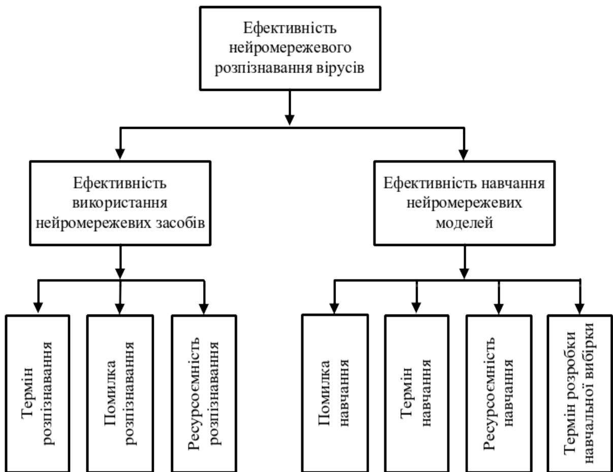
с. 2.4. Показники оцінки ефективності нейромережевого розпізнавання
