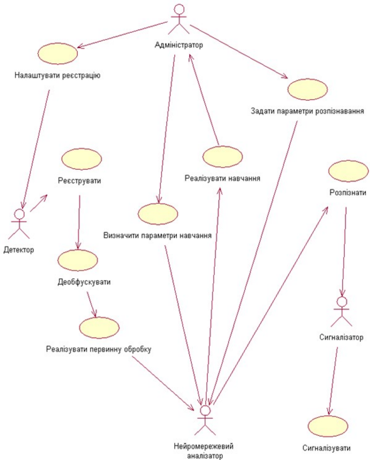
Рис. 4.1. Діаграма прецендентів
