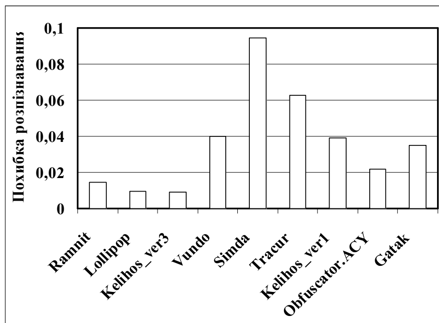
Рис. 4.13. Похибка розпізнавання
